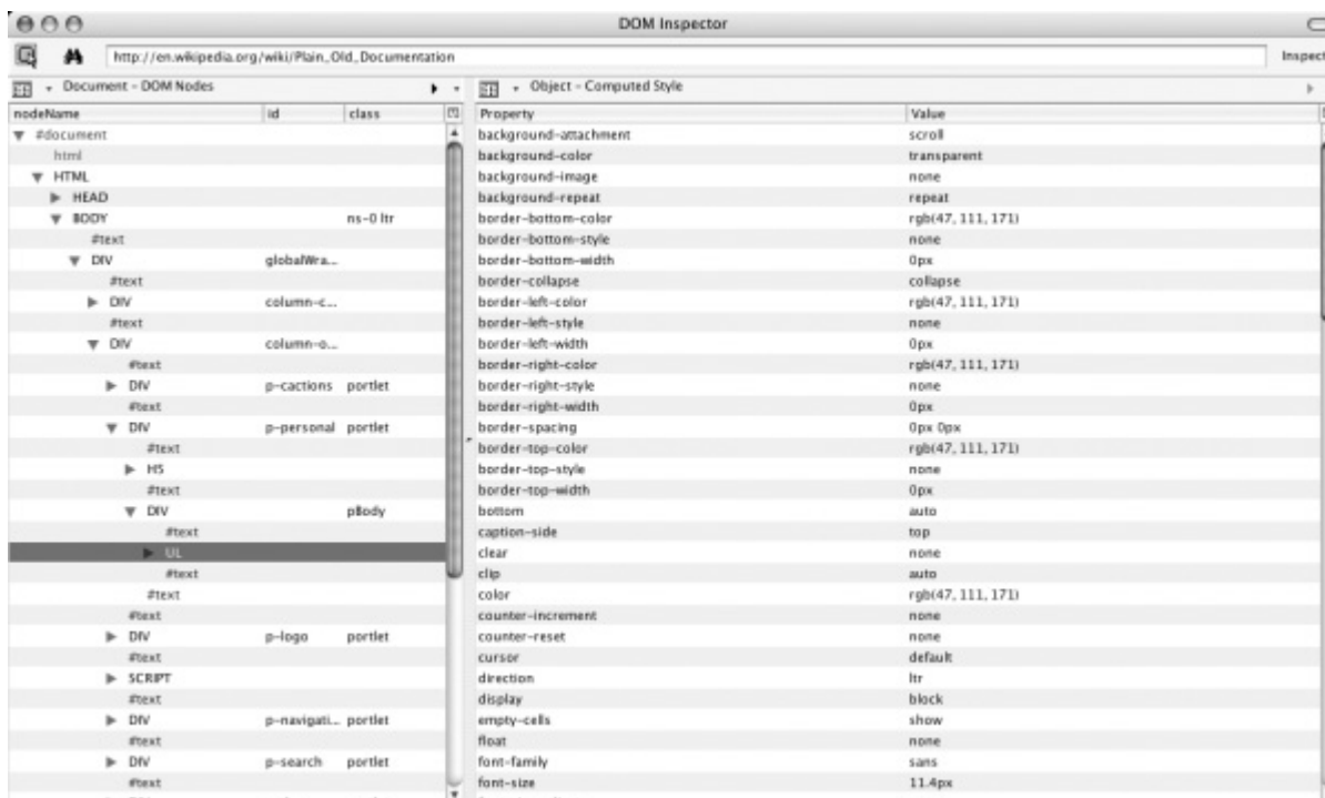
Рис. 4.5. Встроенный в Firefox DOM-инспектор
